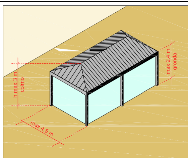
Struttura non appoggiata a parete, con pianta rettangolare e copertura a padiglione. La superficie massima consentita è di 30 mq.
